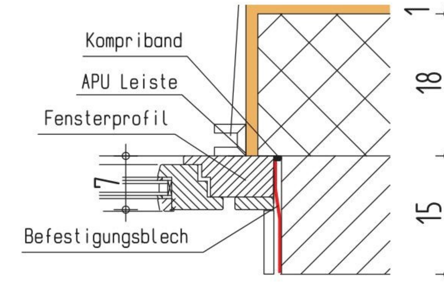
Schnitt Fenster M. 1:5
